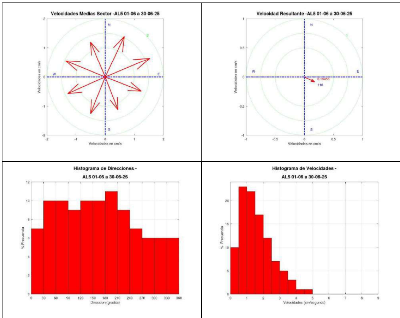
Gráfica 58. Medidas de la dirección y velocidad de la corriente. Vectores e histograma.
