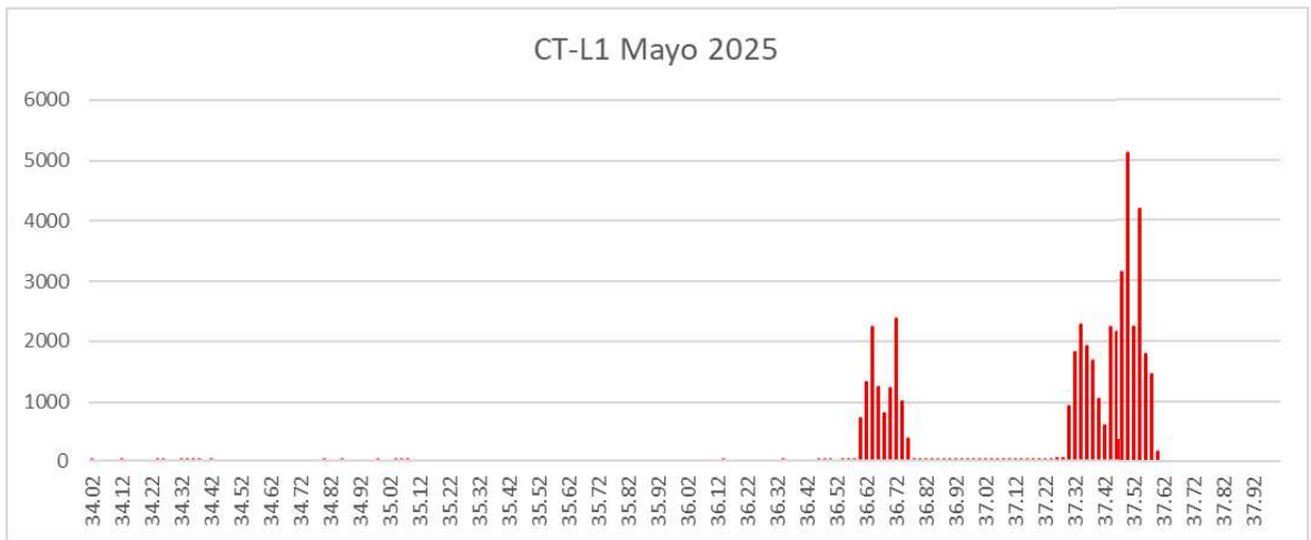
Gráfica 33. Medidas de la salinidad mensual. Dispersión e histograma.
