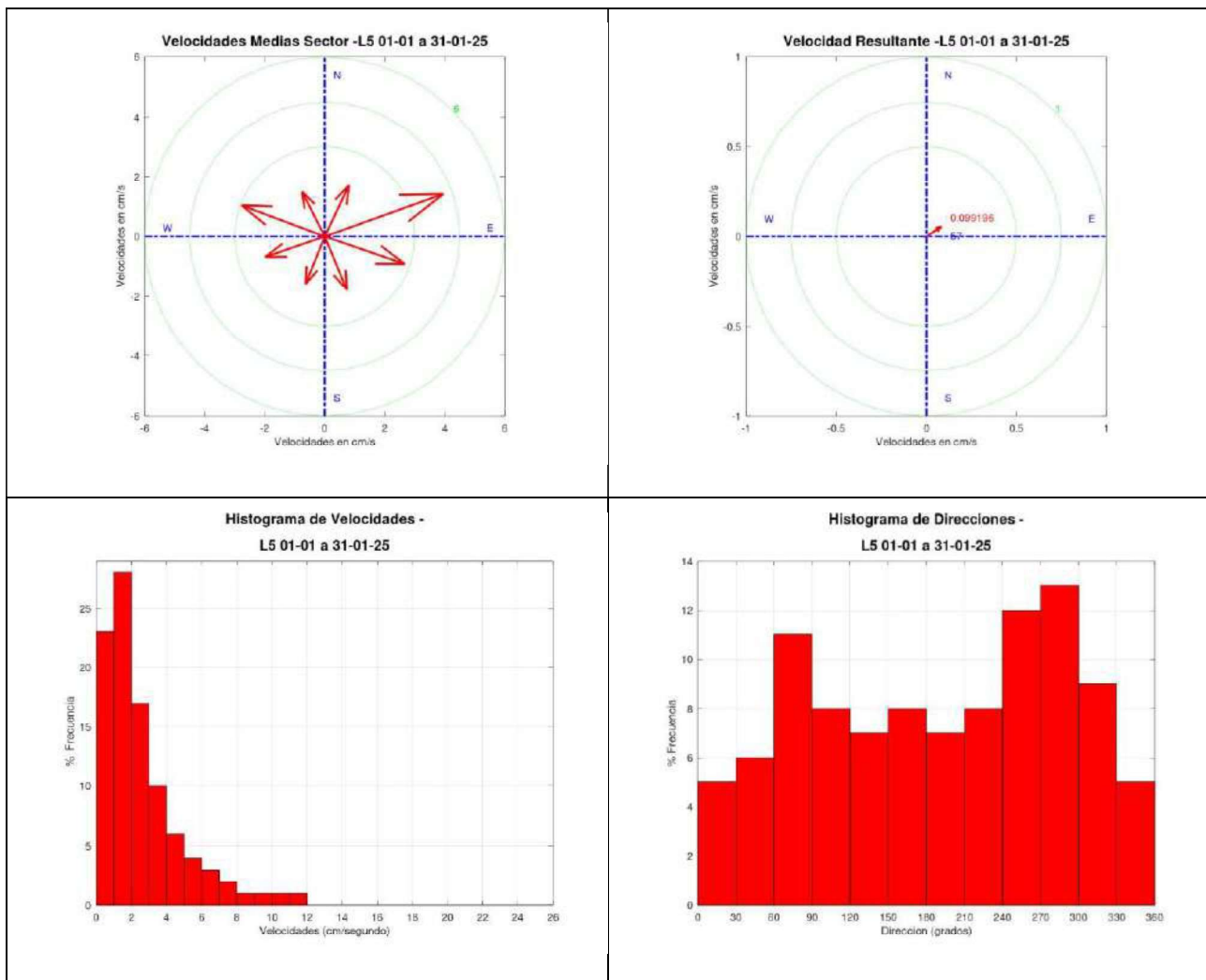
Gráfica 44. Medidas de la dirección y velocidad de la corriente. Vectores e histograma.
