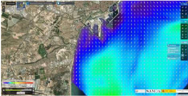
Figura 14. Detalle vector de corriente de componente norte. Entorno de Alicante. 2025
