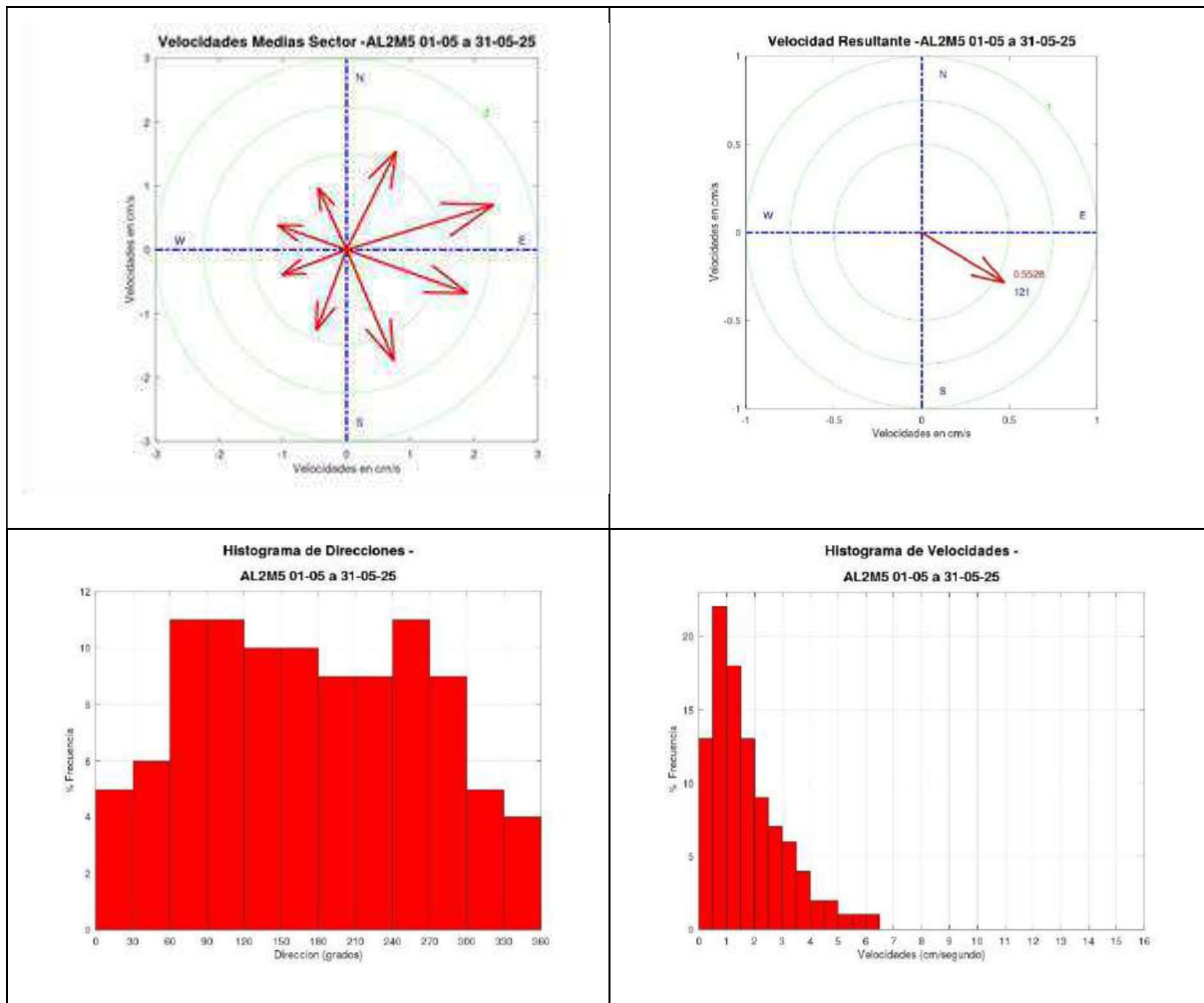
Gráfica 53. Medidas de la dirección y velocidad de la corriente. Vectores e histograma.
