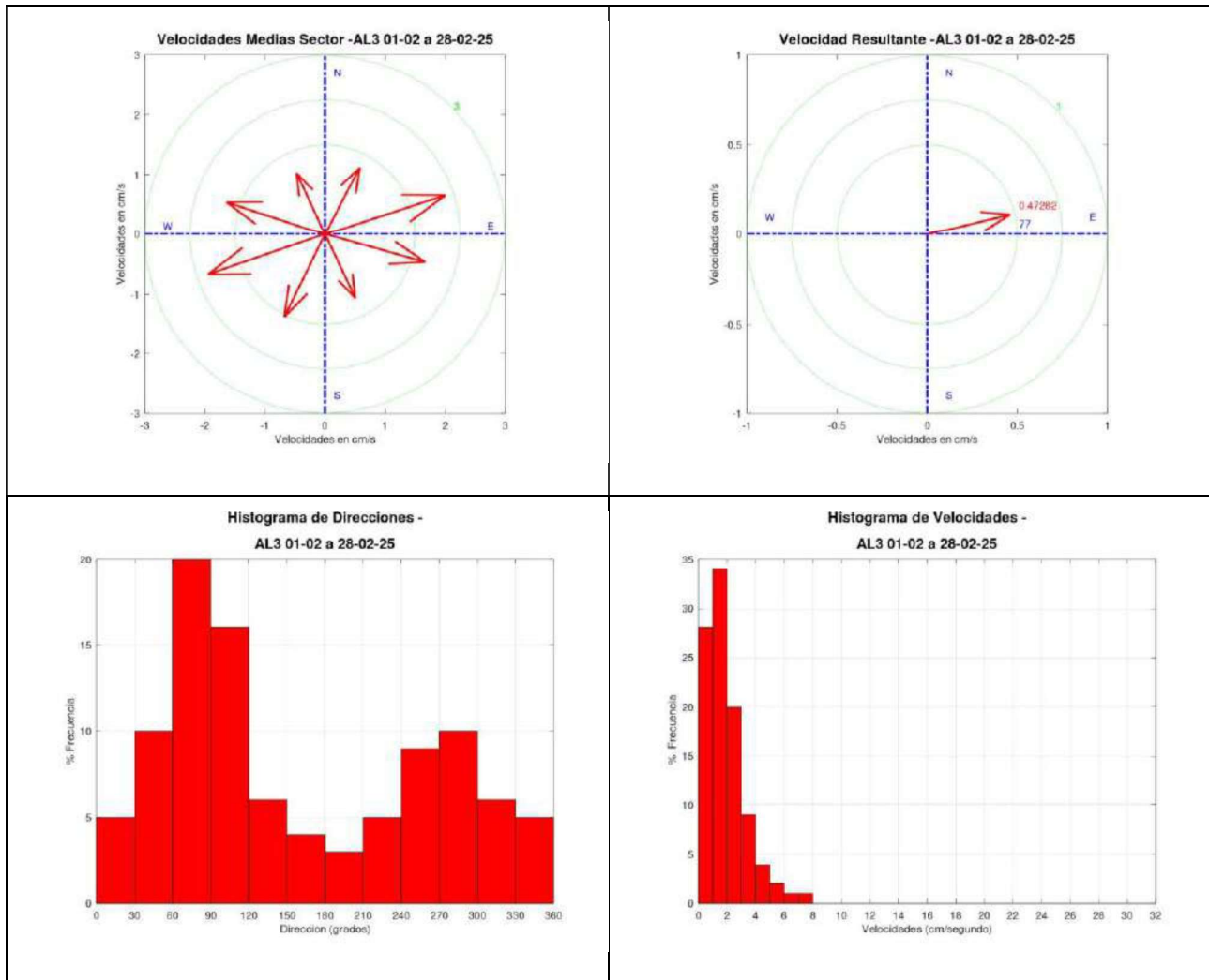
Gráfica 46. Medidas de la dirección y velocidad de la corriente. Vectores e histograma.
