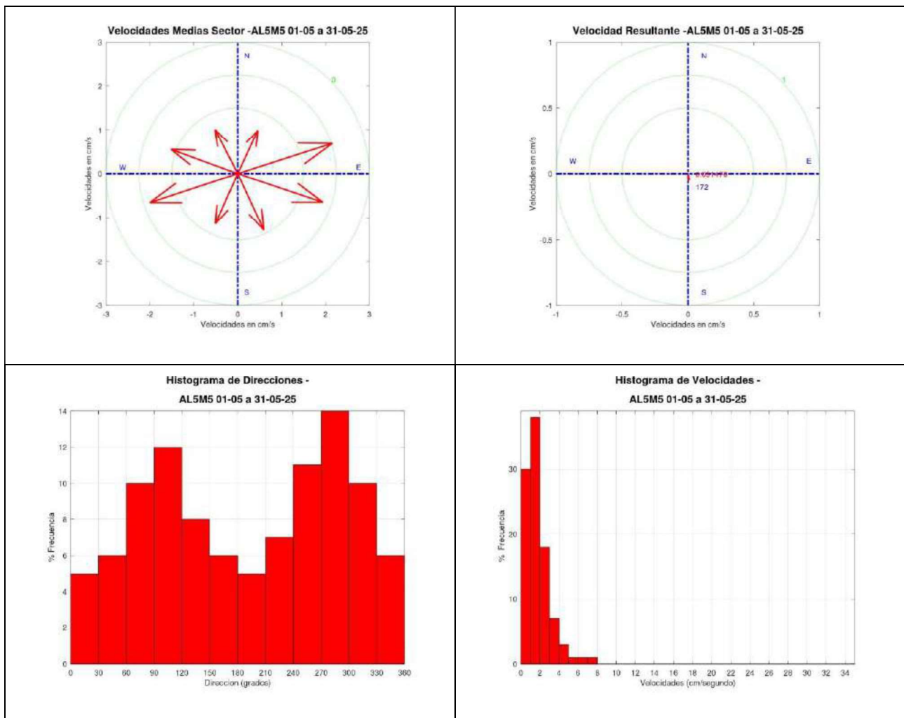
Gráfica 55. Medidas de la dirección y velocidad de la corriente. Vectores e histograma.
