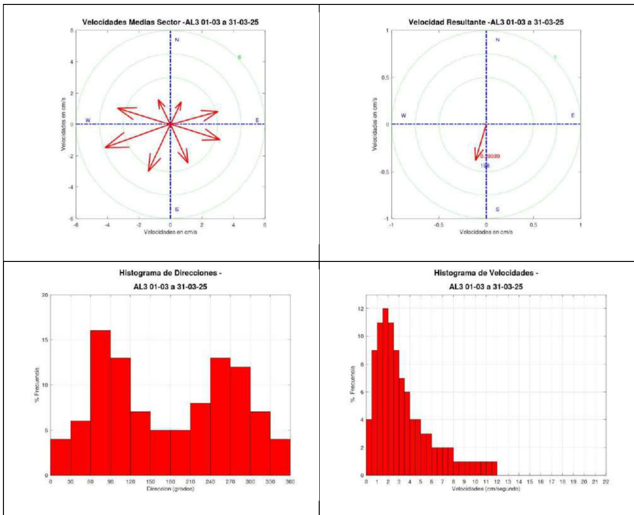
Gráfica 49. Medidas de la dirección y velocidad de la corriente. Vectores e histograma.
