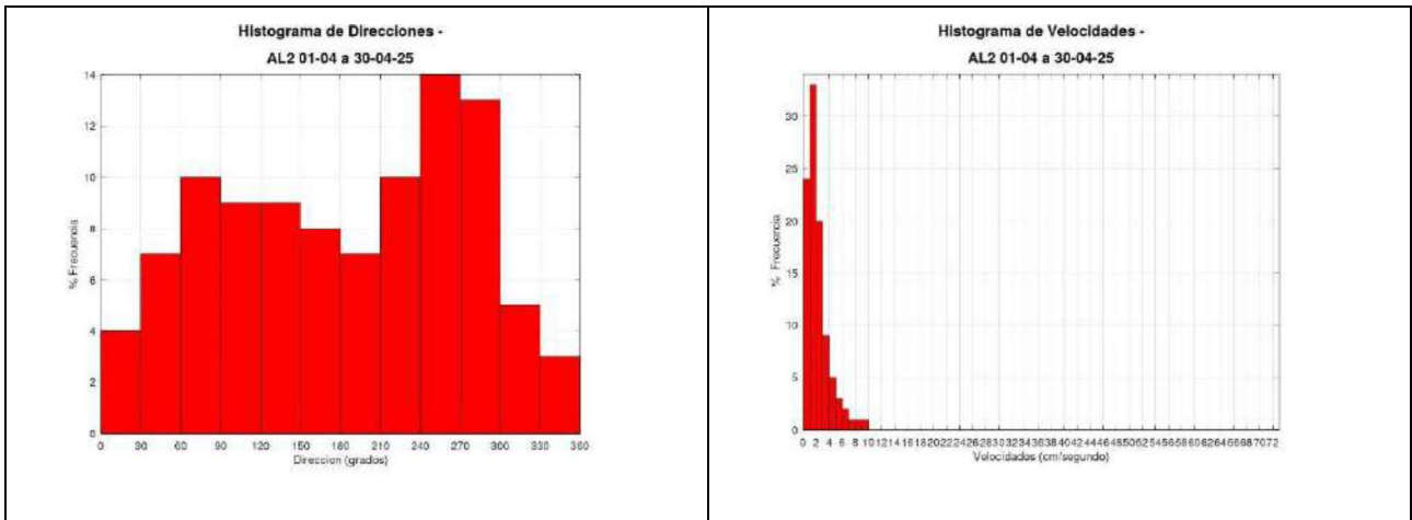
Gráfica 51. Medidas de la dirección y velocidad de la corriente. Vectores e histograma.
