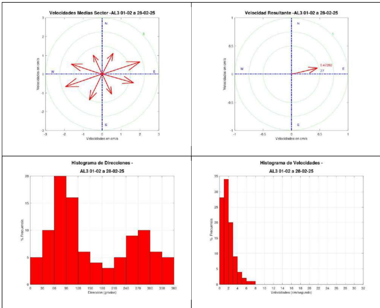
Gráfica 54. Medidas de la dirección y velocidad de la corriente. Vectores e histograma.
