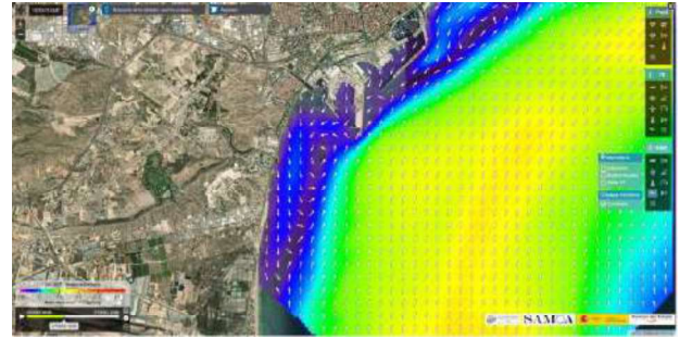
Figura 15. Detalle vector de corriente de componente sur. Entorno de Alicante. 2025
