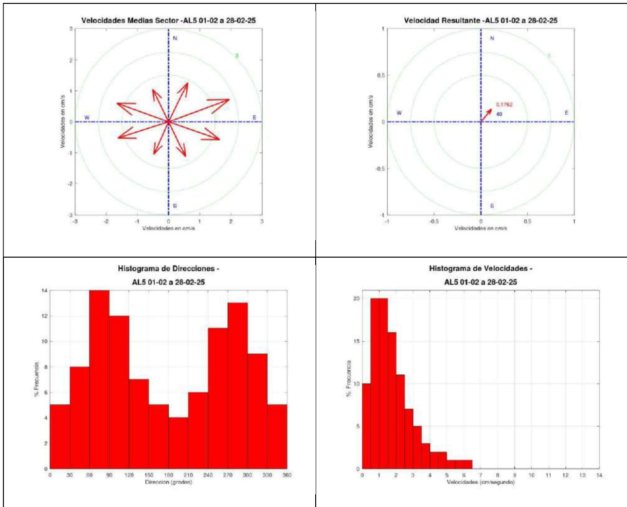
Gráfica 47. Medidas de la dirección y velocidad de la corriente. Vectores e histograma.
