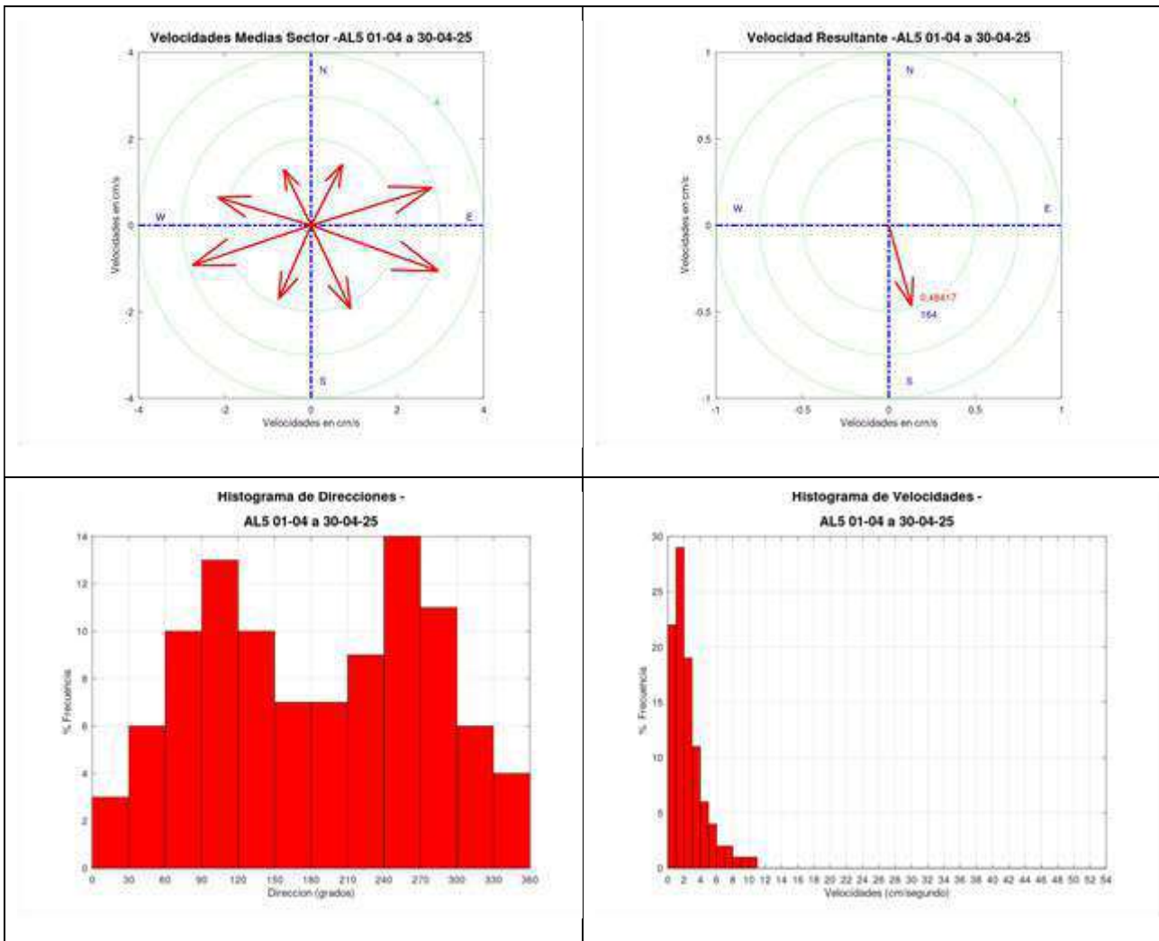
Gráfica 52. Medidas de la dirección y velocidad de la corriente. Vectores e histograma.
