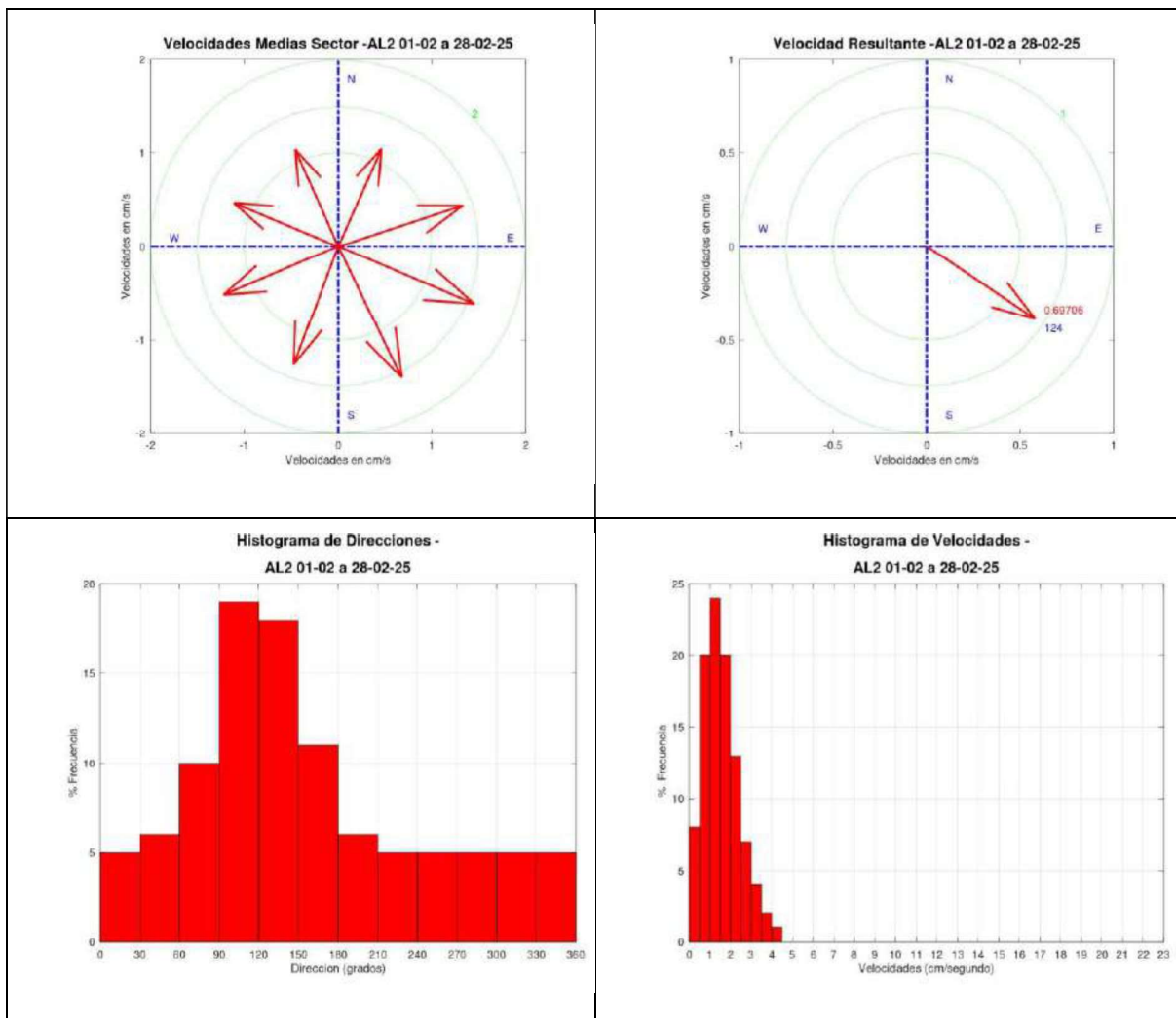
Gráfica 45. Medidas de la dirección y velocidad de la corriente. Vectores e histograma.
