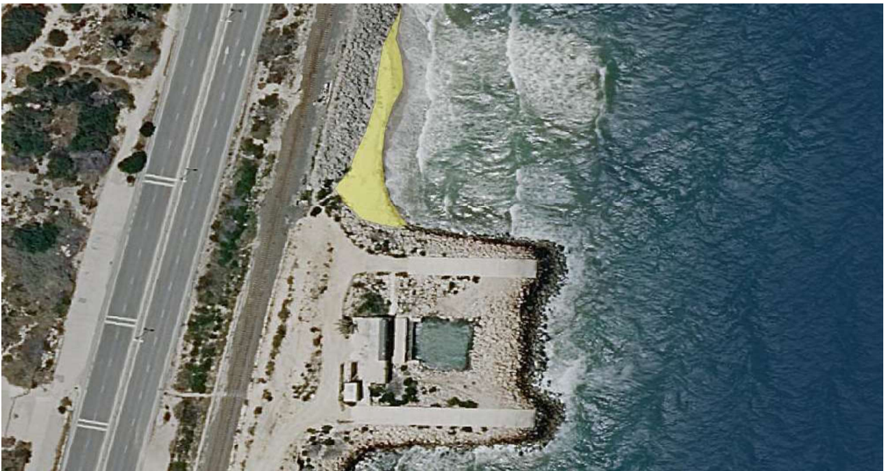
Figura 16. Detalle acumulación de arenas al norte de la estructura asociada a la captación de agua de mar.
