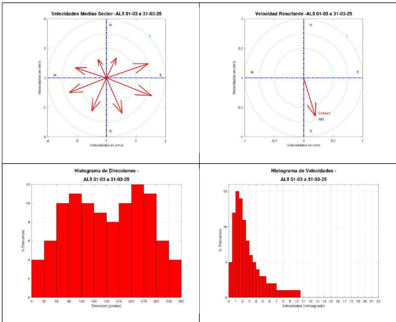
Gráfica 50. Medidas de la dirección y velocidad de la corriente. Vectores e histograma.
