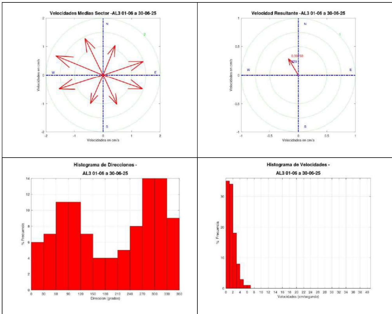
Gráfica 57. Medidas de la dirección y velocidad de la corriente. Vectores e histograma.
