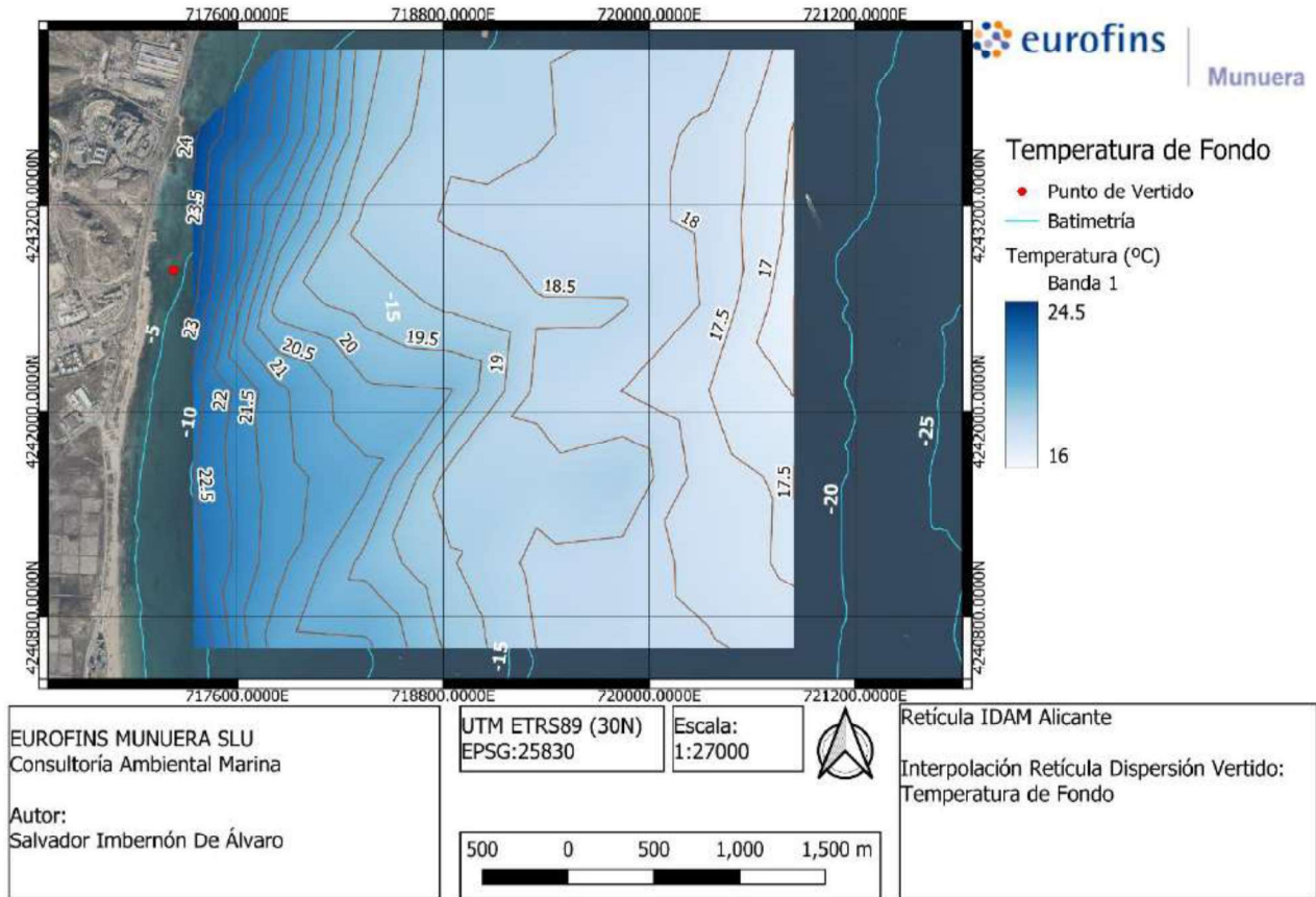
Mapa 9. Interpolación de la retícula de dispersión de la temperatura en el fondo.
