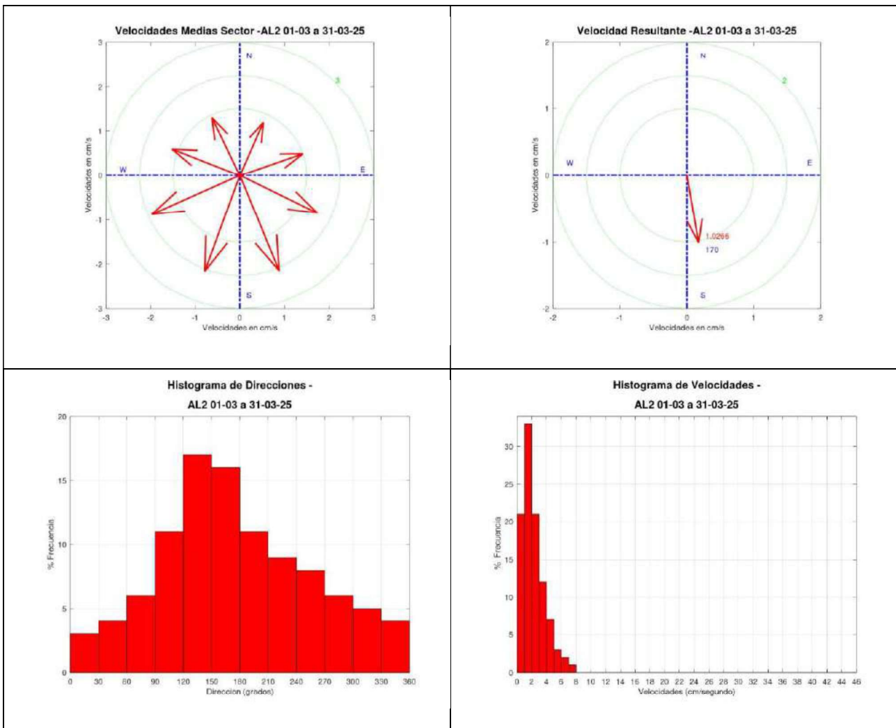
Gráfica 48. Medidas de la dirección y velocidad de la corriente. Vectores e histograma.
