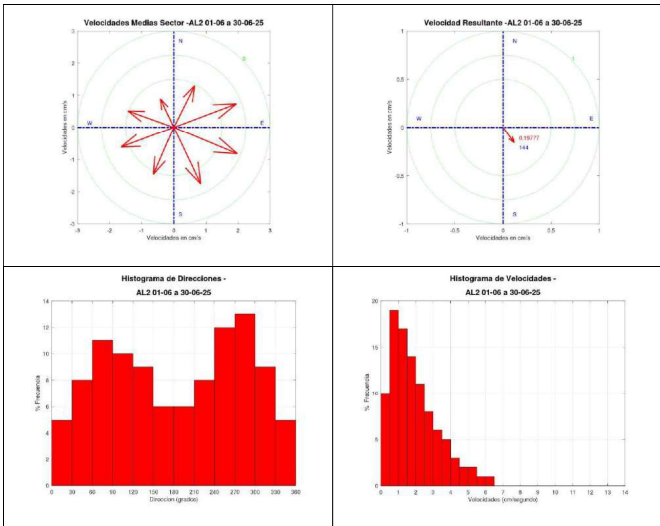
Gráfica 56. Medidas de la dirección y velocidad de la corriente. Vectores e histograma.
