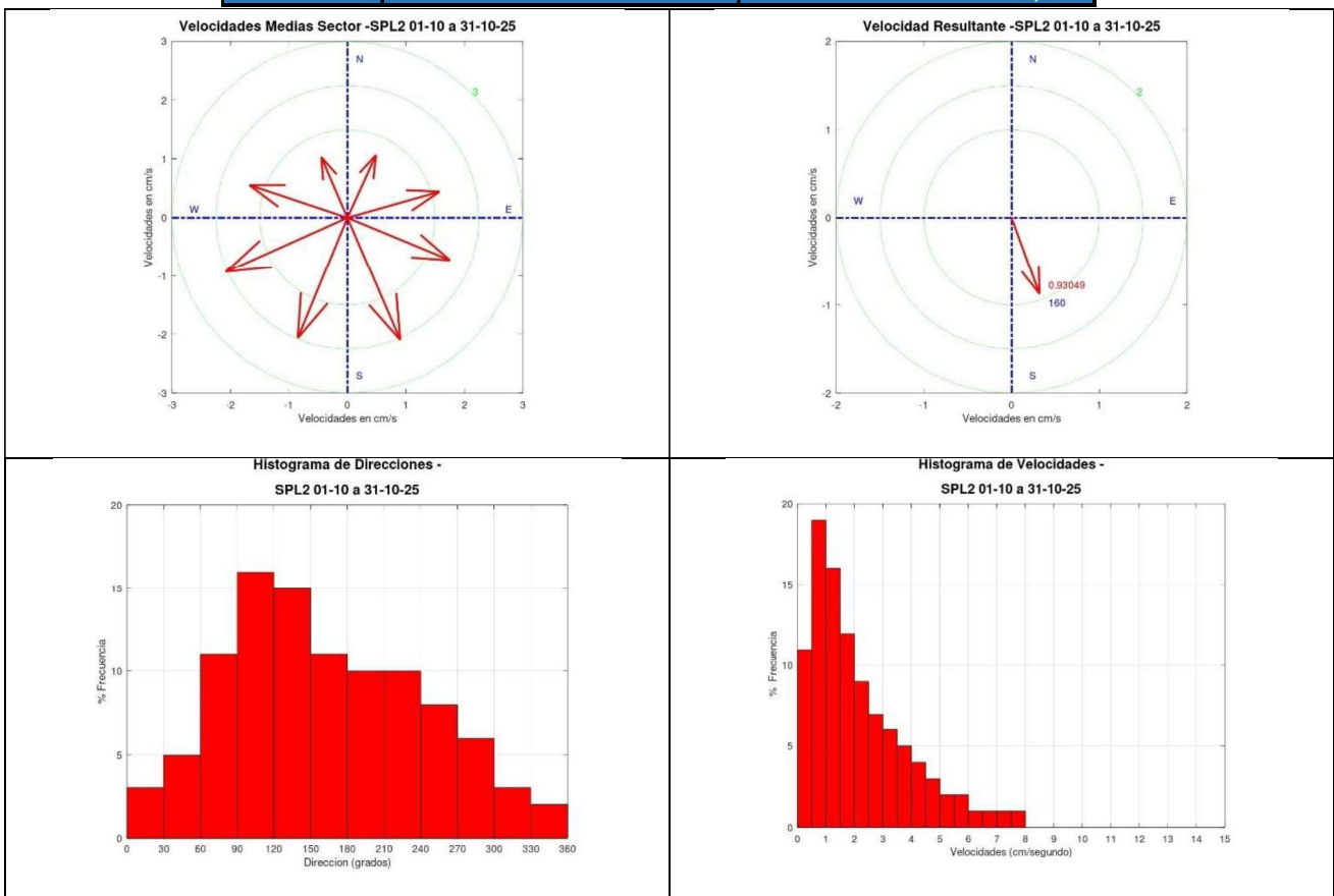
Gráfica 21 Medidas de la dirección y velocidad de la corriente. Vectores e histograma
